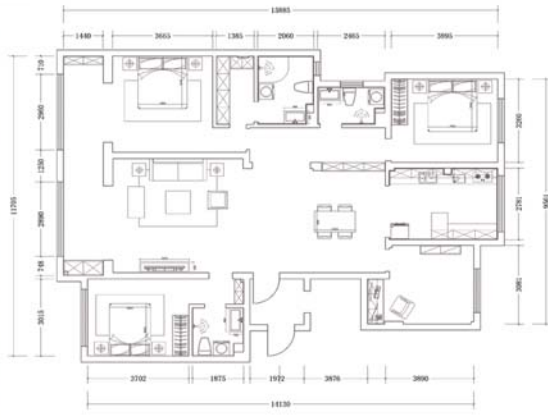
改造后的户型结构图。
