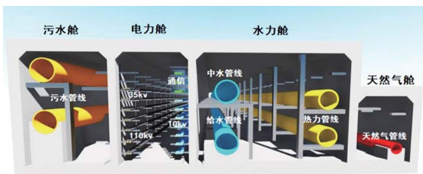
新区地下综合管廊项目贡北路段断面图。
